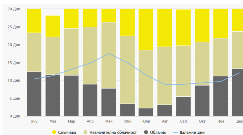
Фигура 3: Облачни, слънчеви и валежни дни в община Симитли. Източник: Meteoblue.
